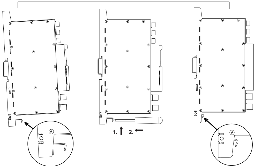
Figure 4. Mounting to DIN rail / Крепление к планке "DIN rail" / Montaggio su barra DIN
